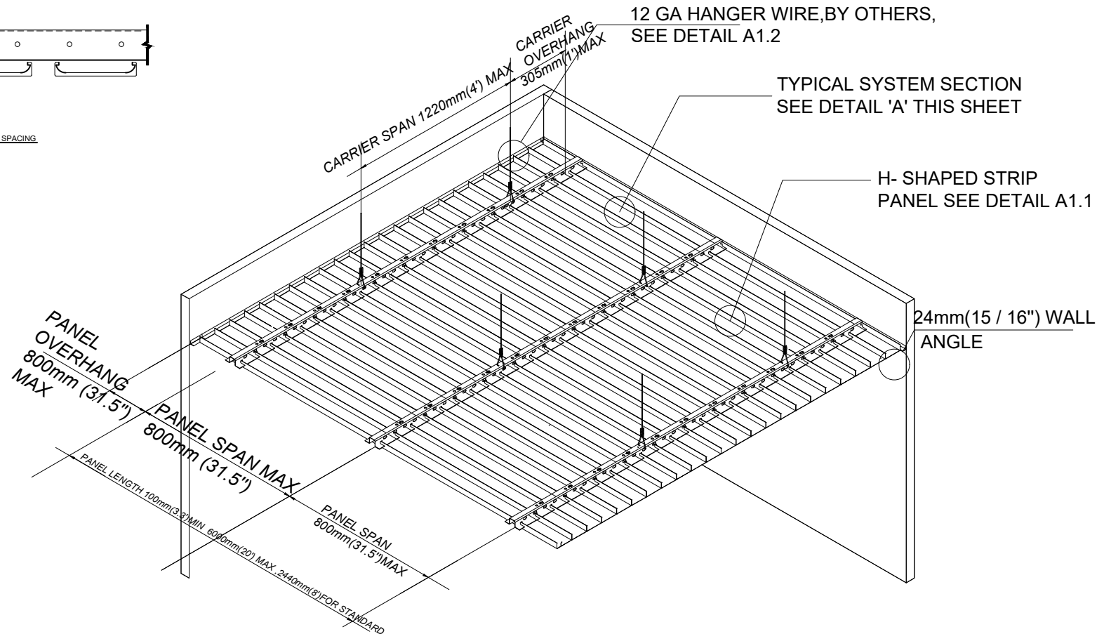
DETAIL 'A' SCALE: 3"=1'-0"
